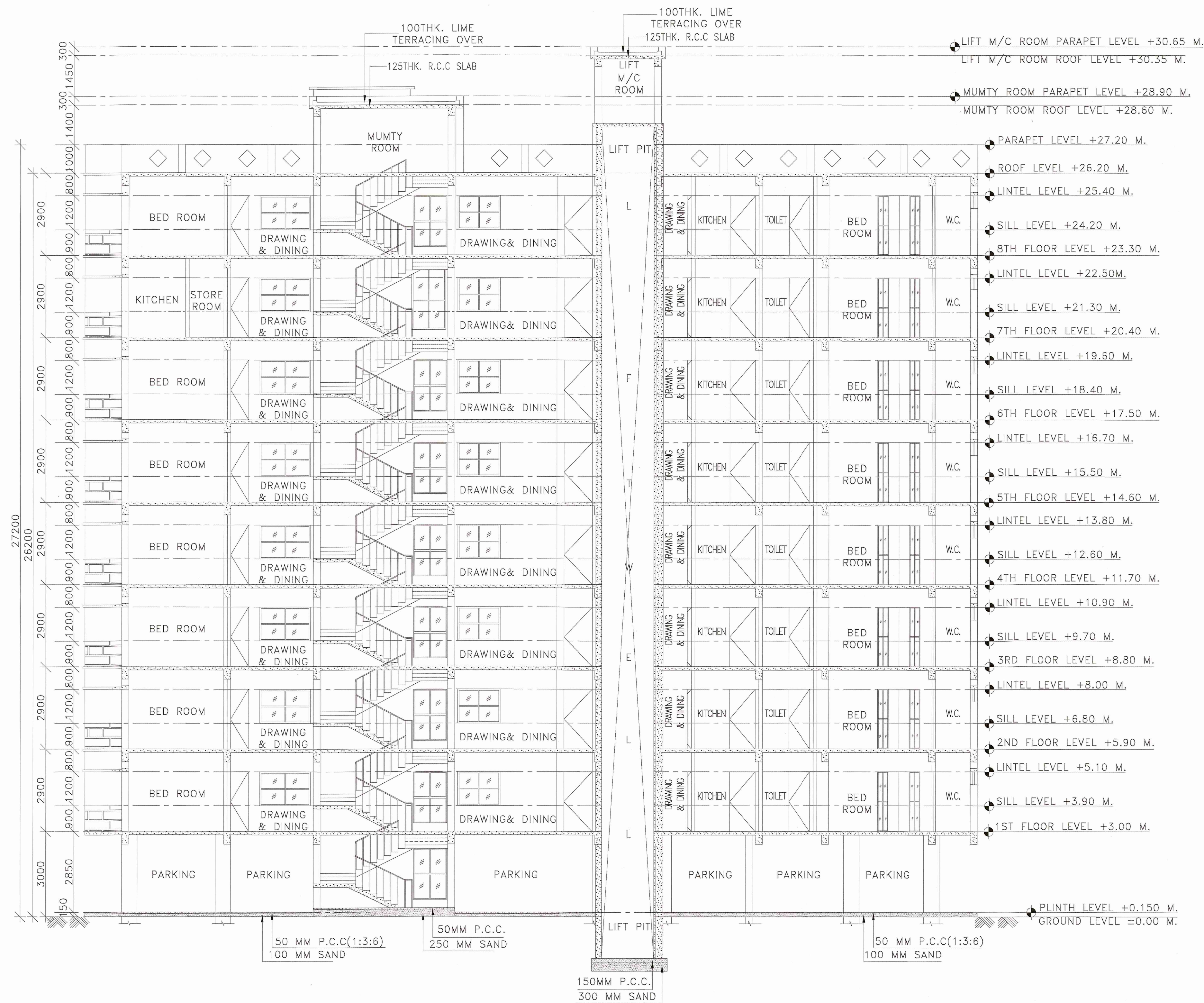
B SECTION Y-Y SCALE: 1:100
